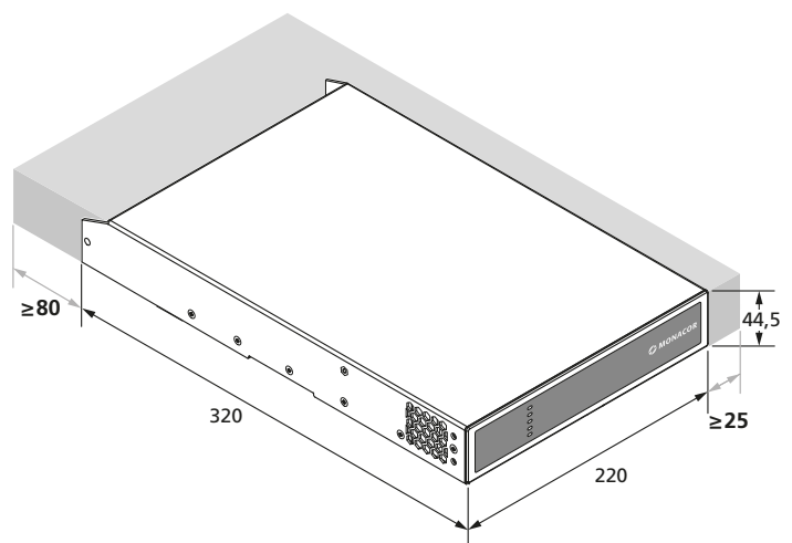
Abb. 4 Belüftungsabstände
