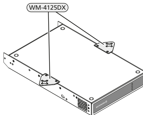
Abb. 8 Montageplatten an Geräteunterseite
