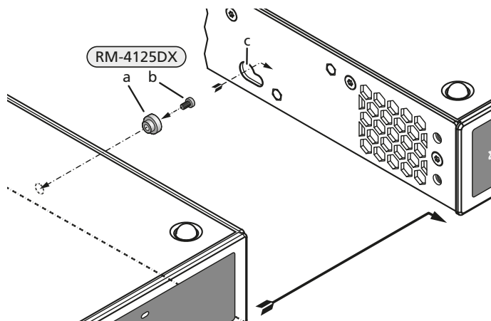
Fig. 6 Installing the stud
