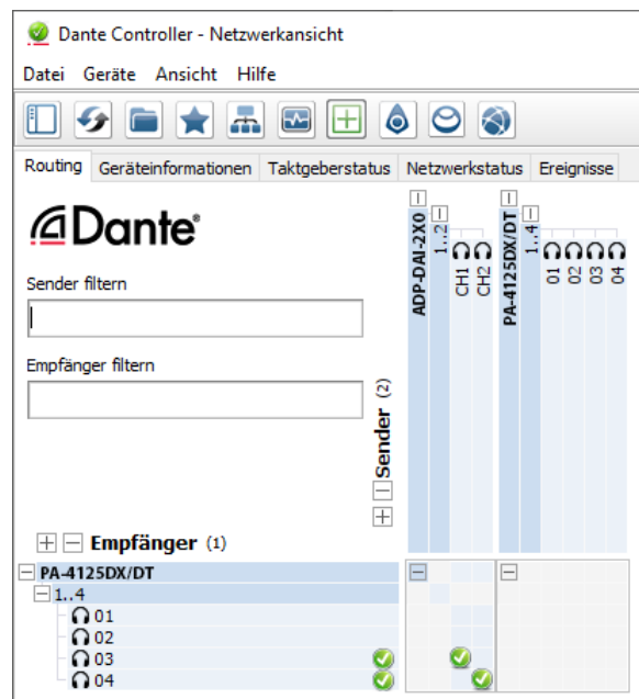
Abb. 38 Routing vom ADP-DAI-2X0 zum PA-4125DX/DT
