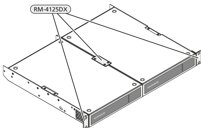
Abb. 7 Verbindungsplatte und Rackmontagewinkel
