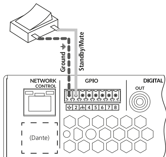
Abb. 11 externer Standby/Mute-Schalter
