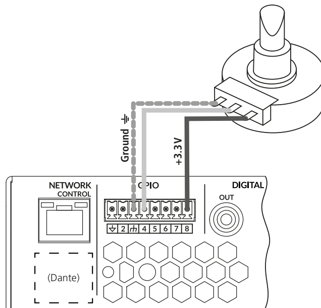
Abb. 10 externer Lautstärkeregler
