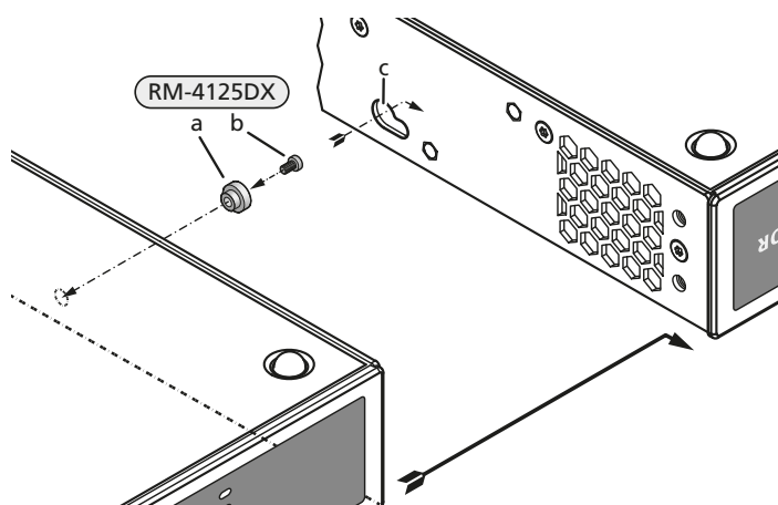
Abb. 6 Montage des Verbindungszapfens
