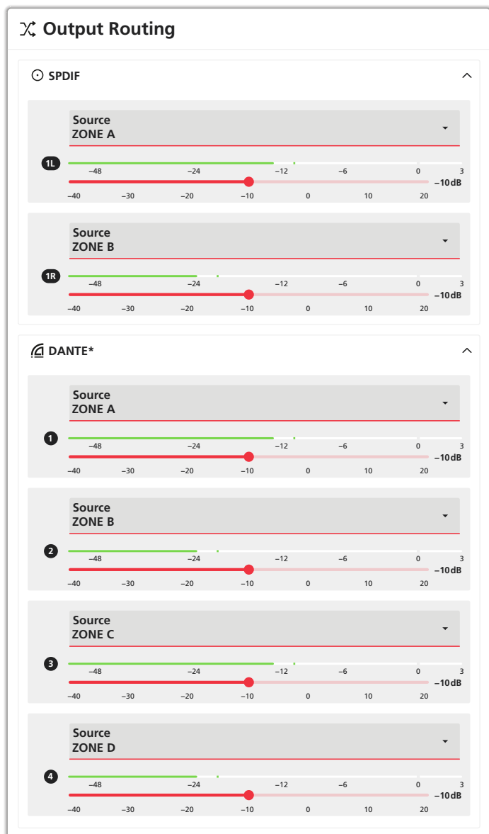
Abb. 35 Ansicht „Output – Speaker Preset – Output Mode“ (* nur bei PA-4125DX/DT)
