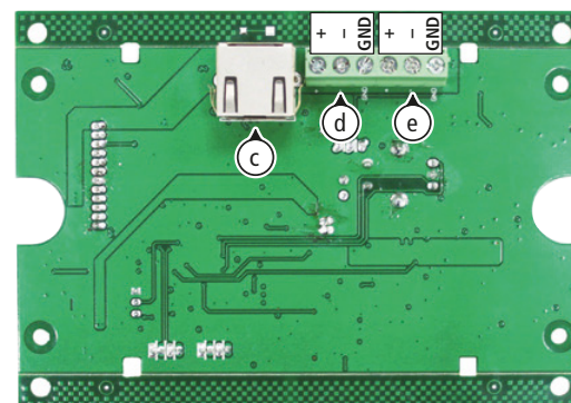
Abb. 6 Anschluss DRM-884VAP
