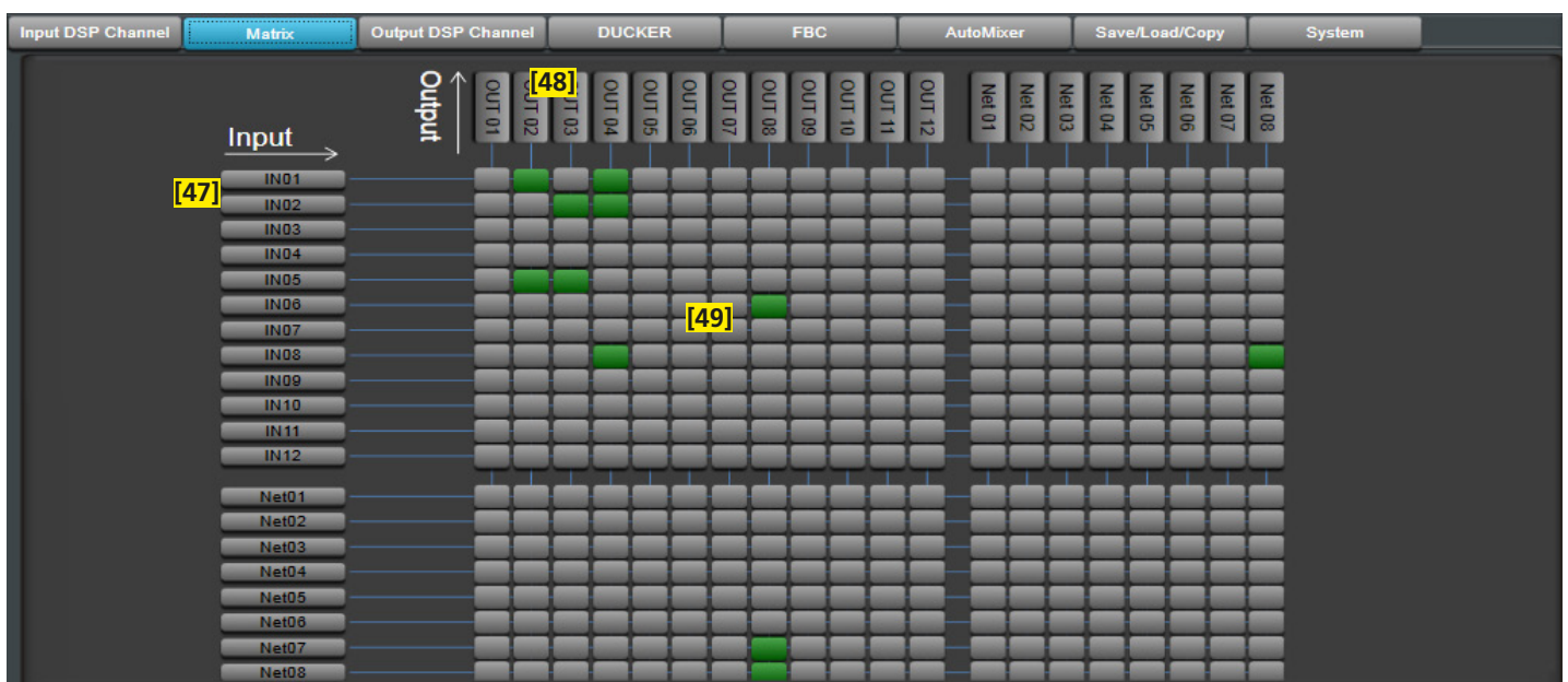
Abb. 21 Ansicht „Matrix“
