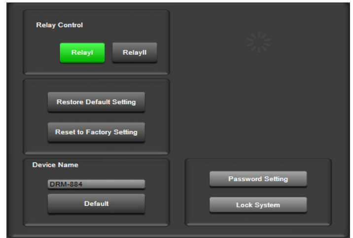
Abb. 29 Ansicht „System“
