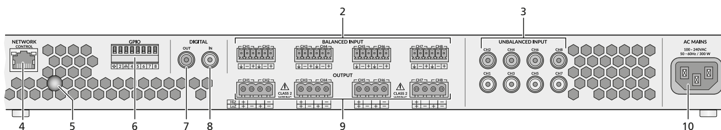
Abb. 3 Rückseite
