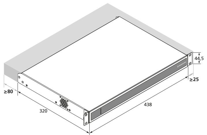
Abb. 4 Belüftungsabstände
