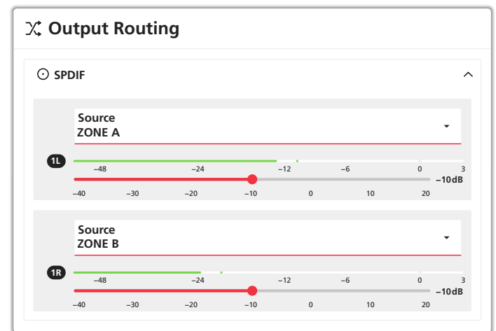
Abb. 30 Ansicht „Output – Speaker Preset – Output Mode“
