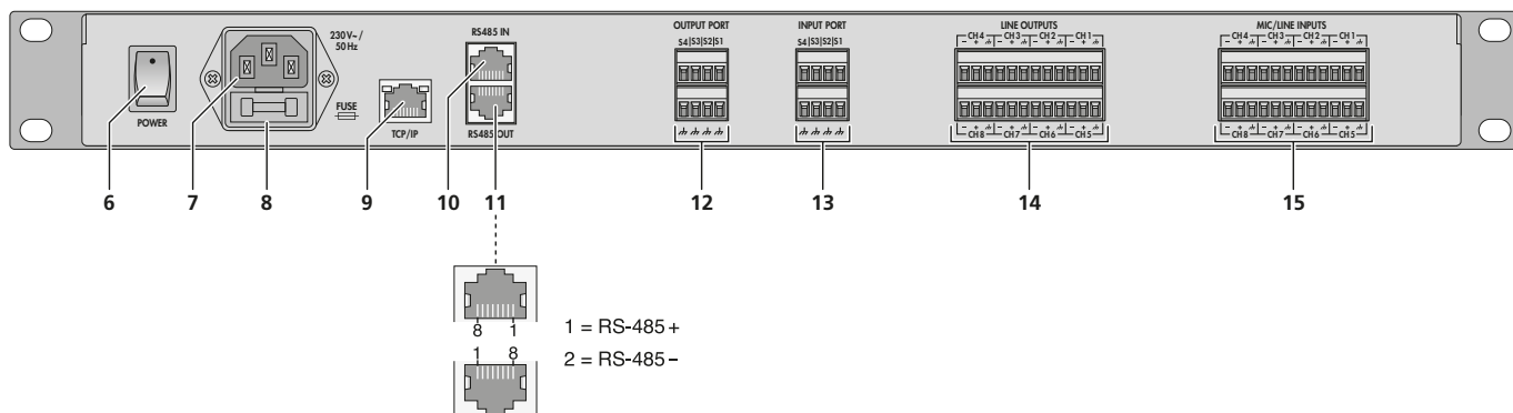
② DRM-882LAN Rückseite • Rear panel
