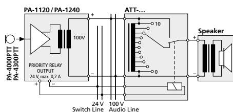
⑥ Relés de prioridad de emergencia
