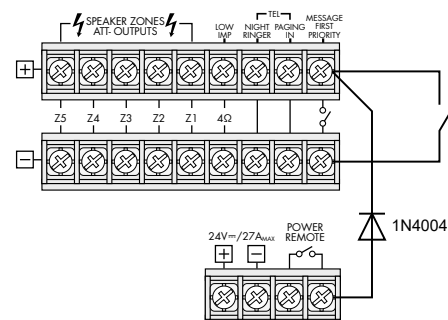
⑦ Automatyczne uruchamianie wzmacniacza i komunikatu z komórki pamięci M 6
