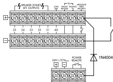
⑦ Conexión automática del amplificador y activación del anuncio M 6
