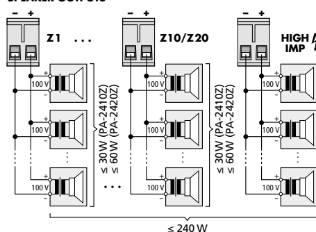
⑧ Collegamenti degli altoparlanti 100V
