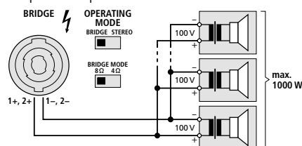
⑥ Funzionamento a 100 V: Le uscite Bridge sono separate galvanicamente dalla rete 230 V e non sono collegate con la massa o la terra.
