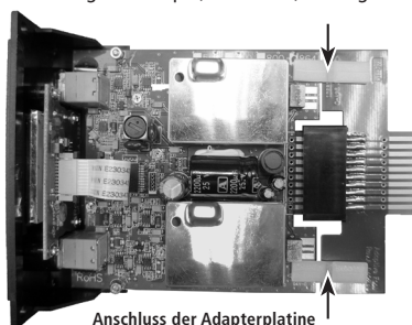
Anschluss der Adapterplatine
