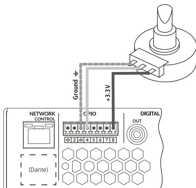
Abb. 4 externer Lautstärkeregler
