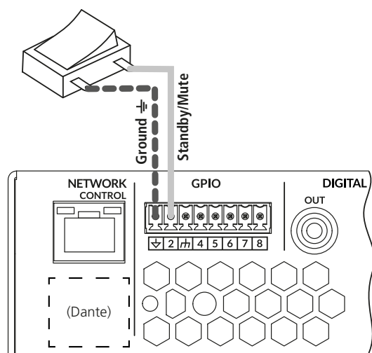
Abb. 5 externer Standby/Mute-Schalter
