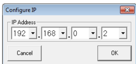
Abb. 15 Auswahl IP-Adresse
