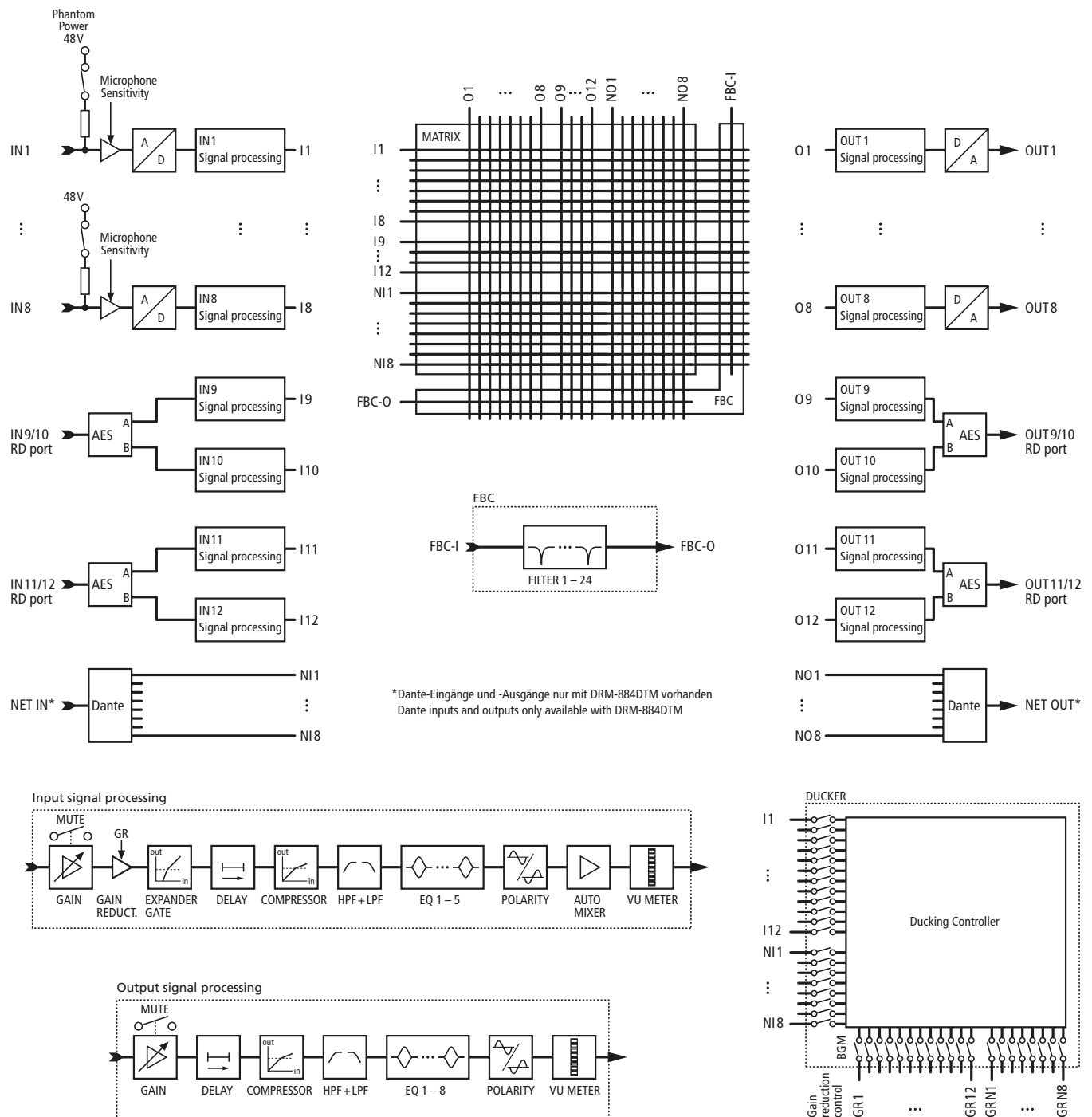
Abb. • Fig. 3 Blockschaltbild • Block diagram
