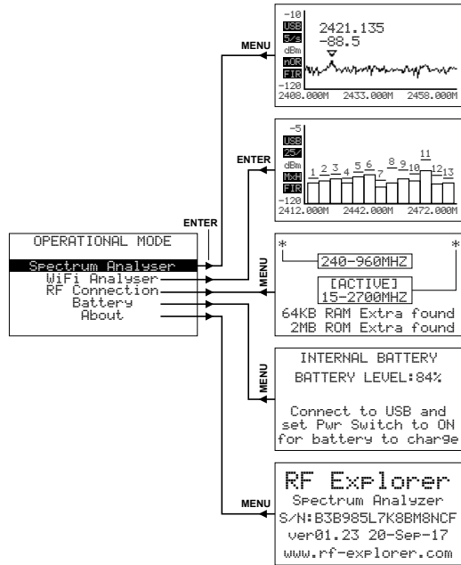
Schéma 5 Operational Mode (Menu mode fonctionnement)
