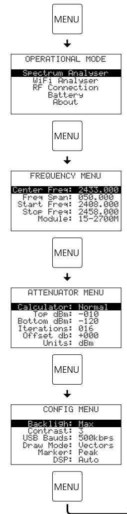
Schéma 4 Structure du menu
