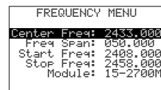
Schéma 6 Menu fréquence
