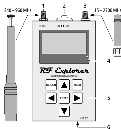
Fig. 1 Collegamento e elementi di comando
