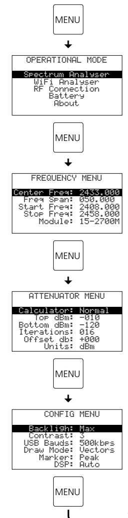
Abb. 4 Menüstruktur
