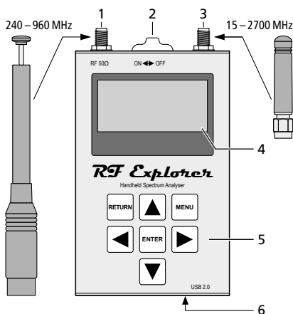
Abb. 1 Anschlüsse und Bedienelemente
